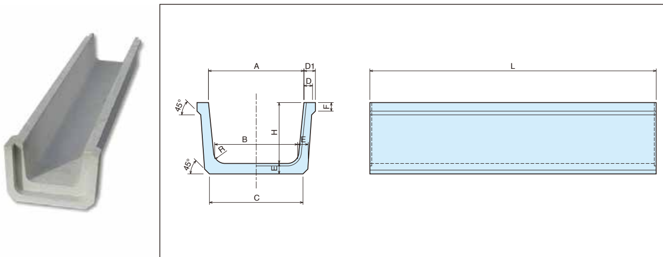
[形状図(ベンチフリュームI種)]
