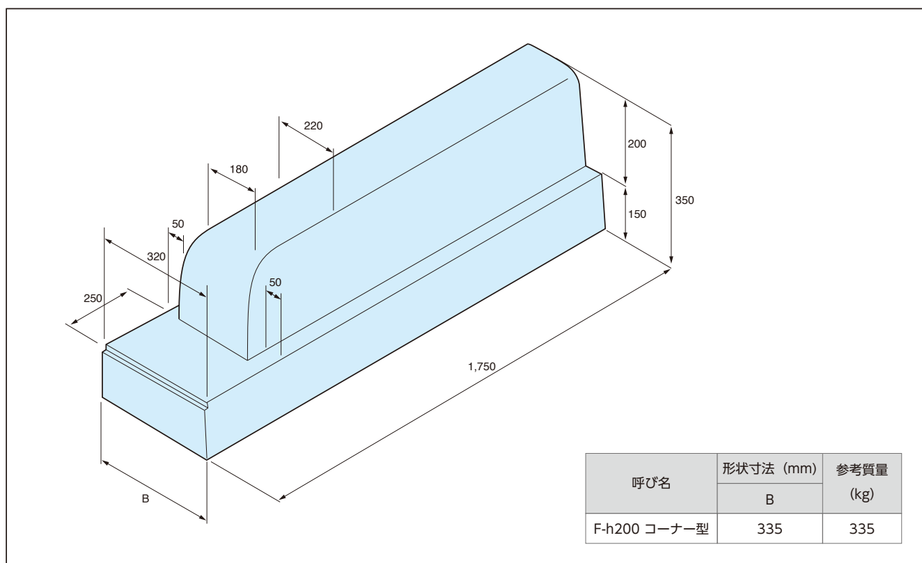
[形状図(フラット・セミフラット コーナー型)]
