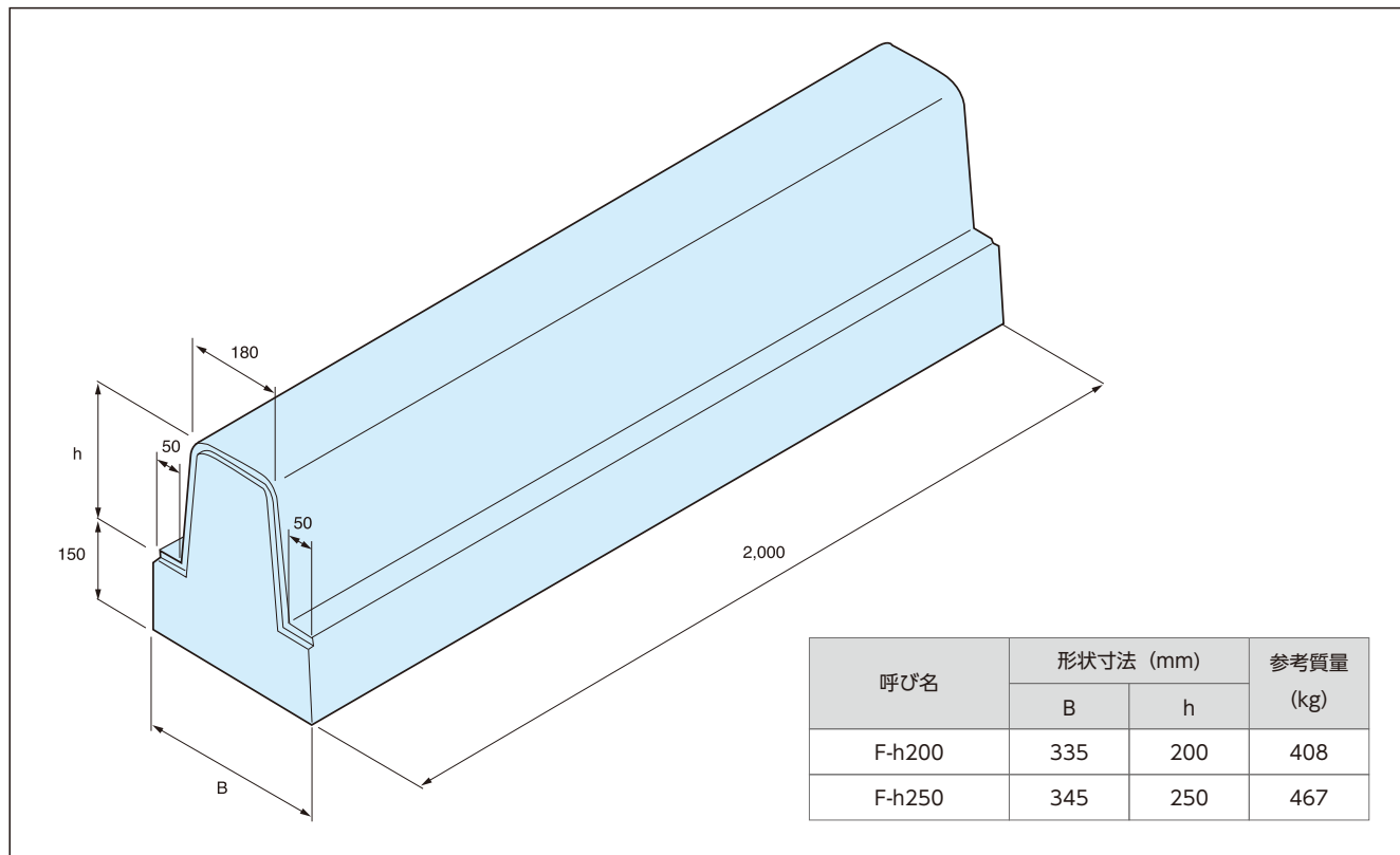
[形状図(フラット・セミフラット 基本型)]
