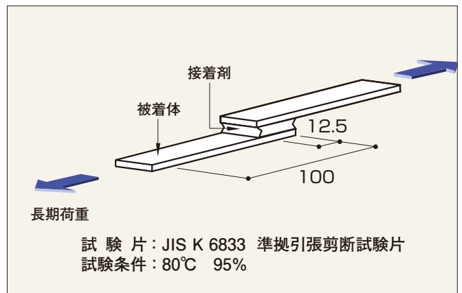
図-1 デッドロードストレス試験概要
